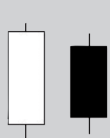
20) Harami (Bearish)
