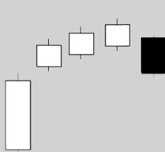
23) Breakaway (Bearish)
